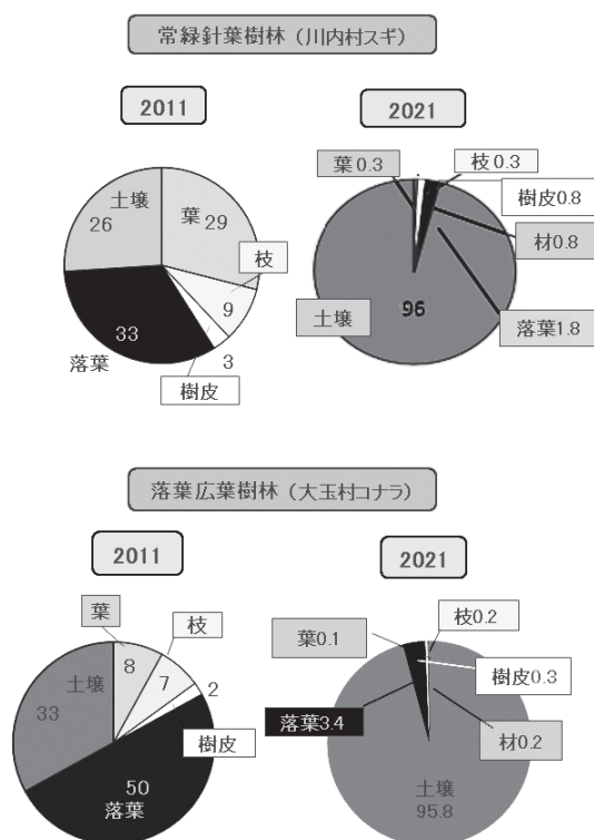
図7. 針葉樹と広葉樹における放射性物質の分布割合 (2022年福島県資料、2022年林野庁資料より)
